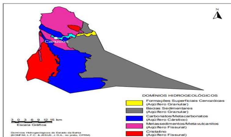
Figura 3: Domínio hidrológico do município
