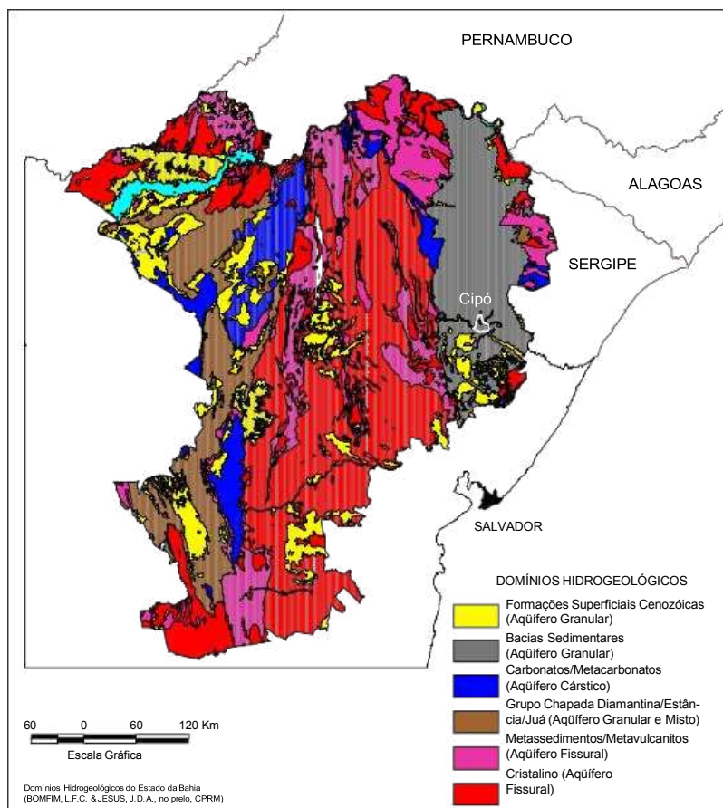
Figura 4 – Domínio hidrogeológico.
