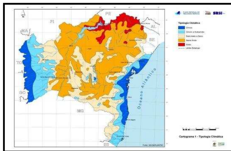
Figura 4: Tipologia Climática na Região. Fonte: Secretaria de Recursos Hídricos (SRH).
