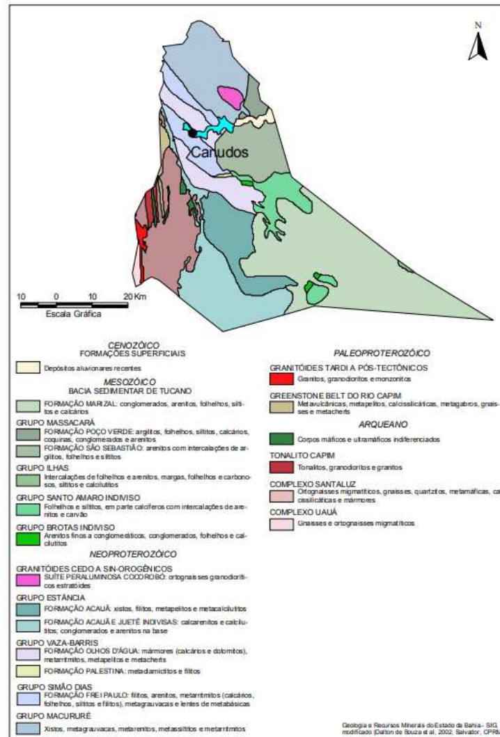
Figura 2: Mapa geológico
